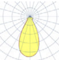
Тип КСС Г, 45°
