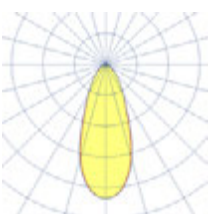
Тип КСС К, 30°
