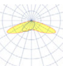
Тип КСС ШБ, 155x70°
