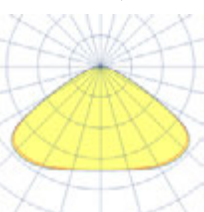
Тип КСС Л, 120°
