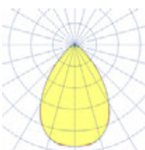
Тип КСС Г, 60°
