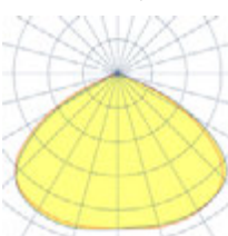
Тип КСС Д, 120°
