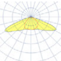
Тип КСС ШБ, 140x85°
