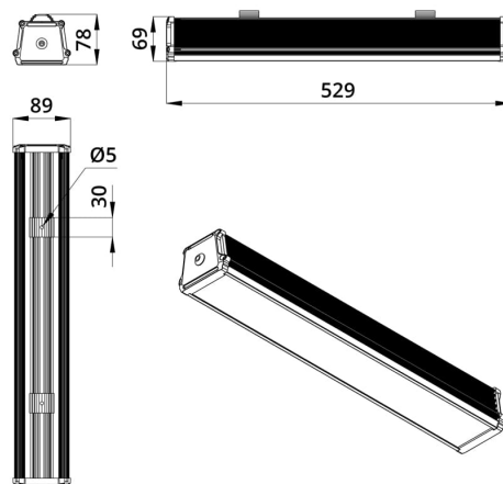
Габаритный чертёж
