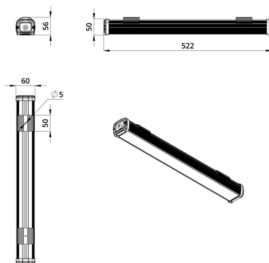
Габаритный чертеж
