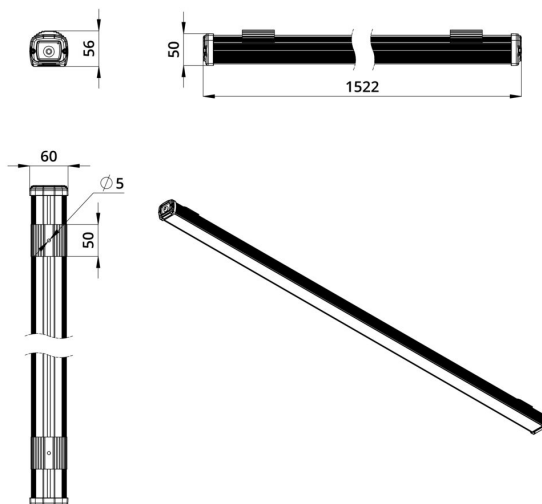
Габаритный чертеж
