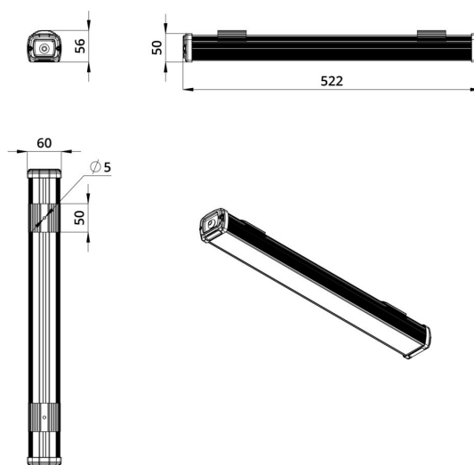
Габаритный чертеж
