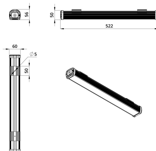
Габаритный чертеж
