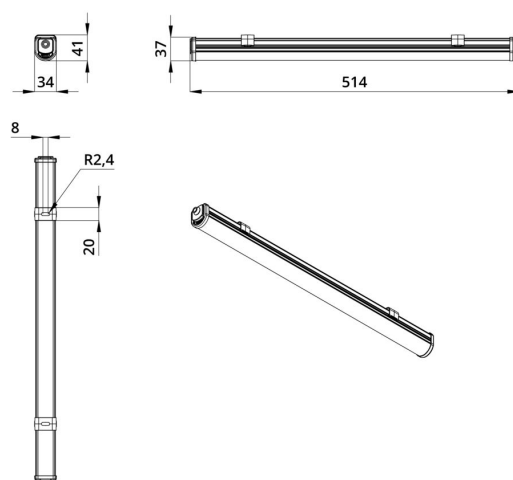
Габаритный чертеж
