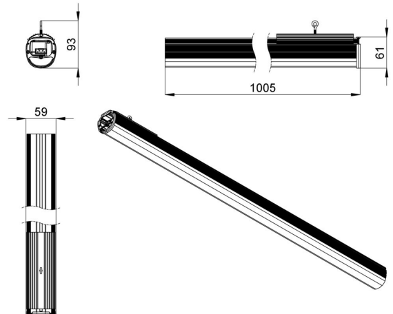
Габаритный чертеж
