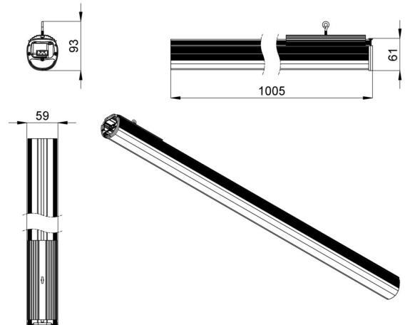
Габаритный чертеж
