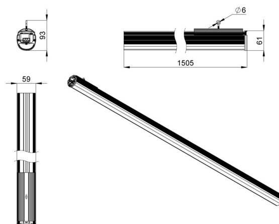
Габаритный чертеж
