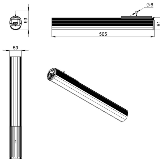
Габаритный чертеж
