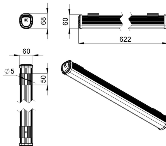
Габаритный чертеж
