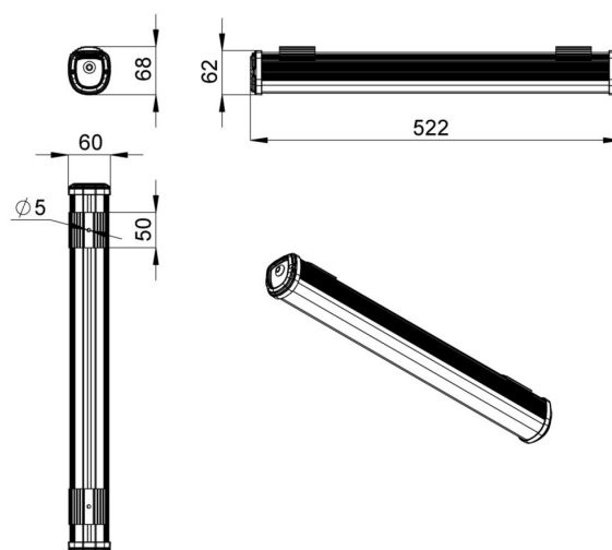
Габаритный чертеж
