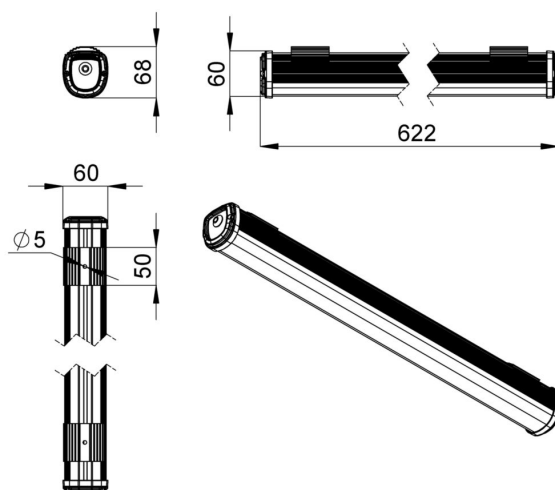
Габаритный чертеж
