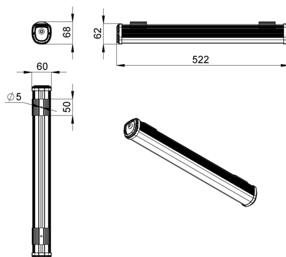
Габаритный чертеж
