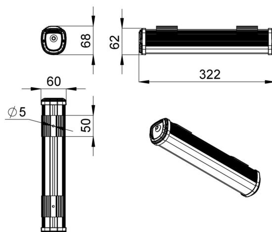
Габаритный чертеж
