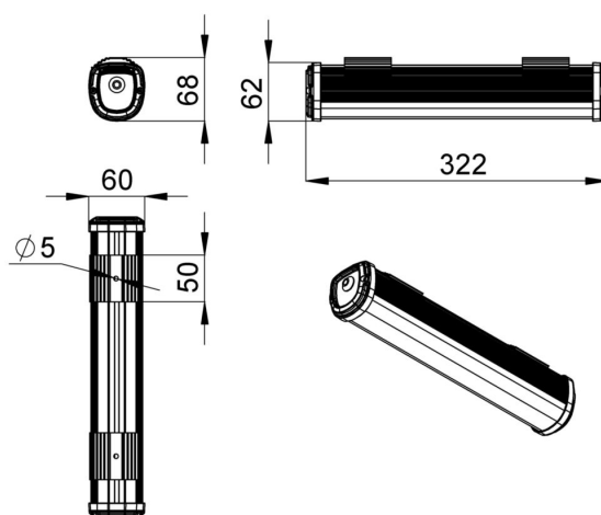
Габаритный чертеж
