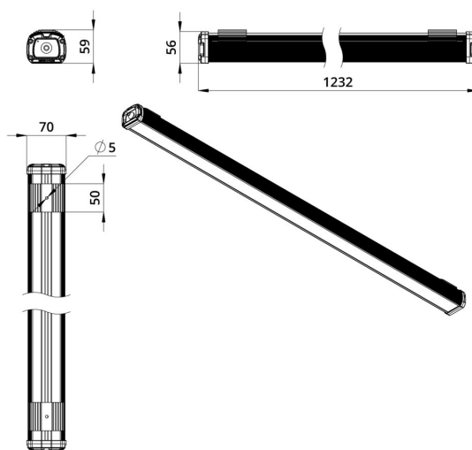
Габаритный чертеж
