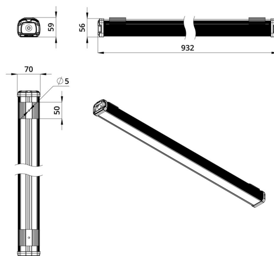
Габаритный чертеж
