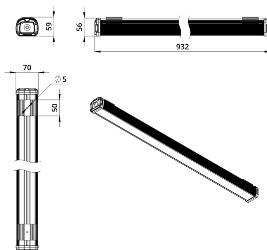
Габаритный чертеж
