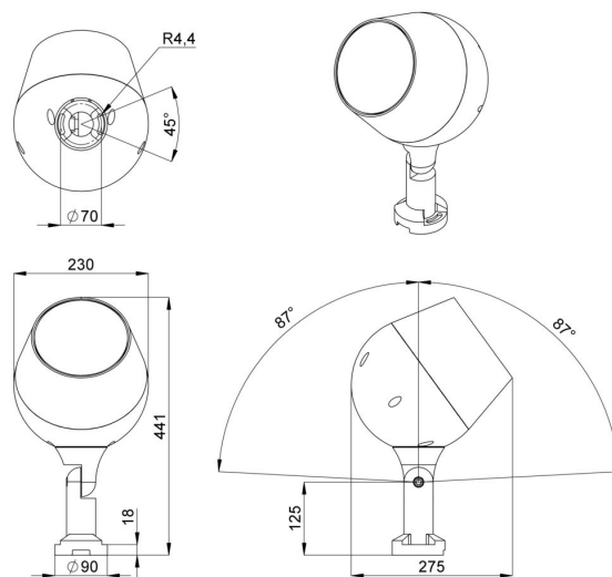
Габаритный чертеж
