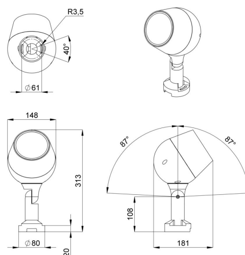
Габаритный чертеж
