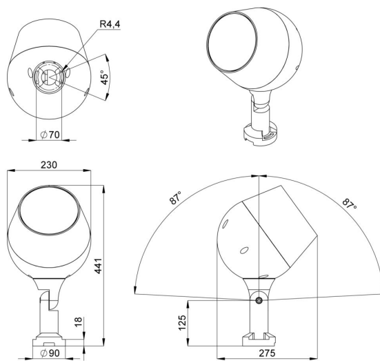
Габаритный чертеж
