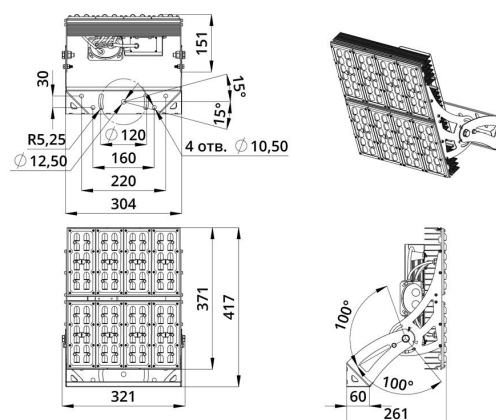
Габаритный чертеж
