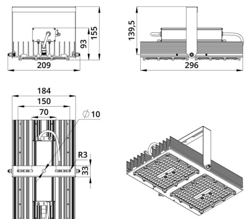
Габаритный чертеж
