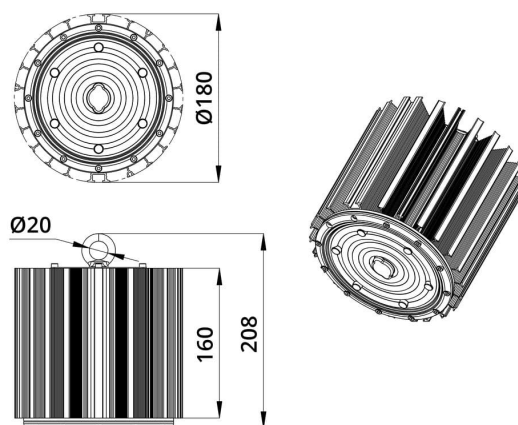
Габаритный чертеж
