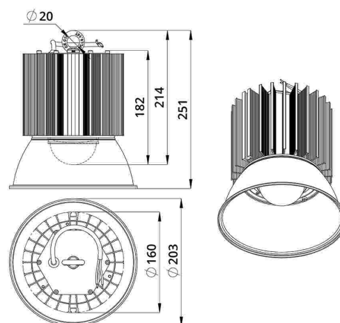
Габаритный чертеж
