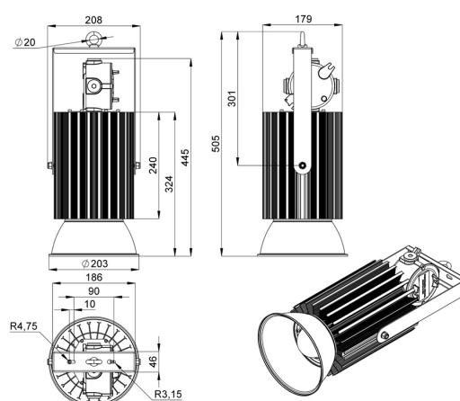
Габаритный чертеж
