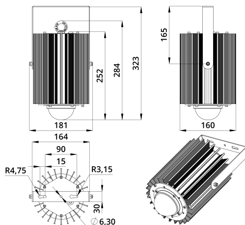
Габаритный чертеж
