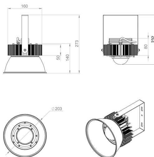
Габаритный чертёж
