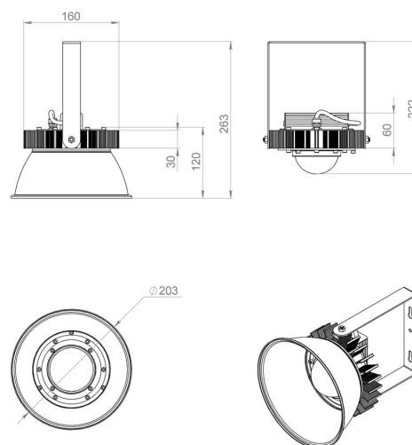
Габаритный чертеж
