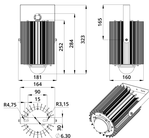
Габаритный чертеж
