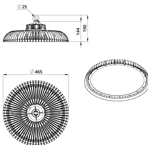
Габаритный чертеж
