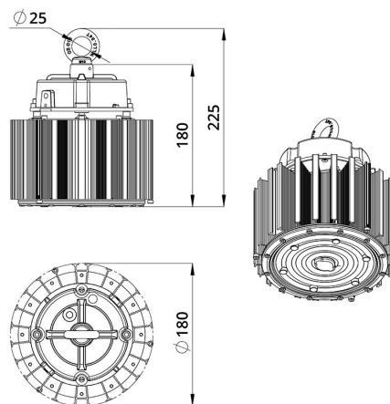
Габаритный чертеж
