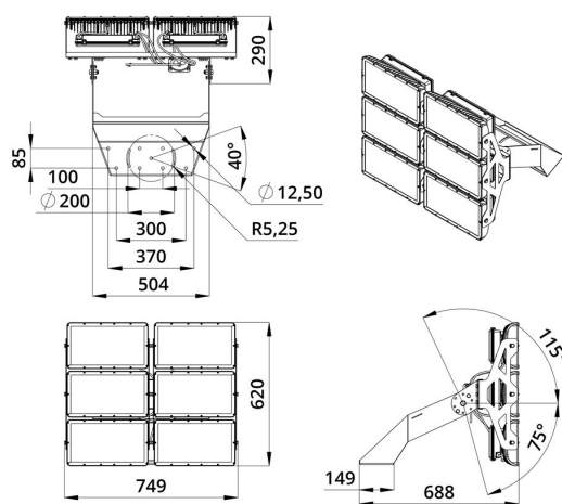
Габаритный чертеж
