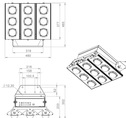
Габаритный чертеж
