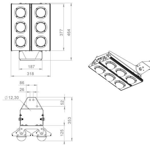
Габаритный чертеж
