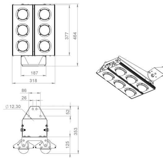
Габаритный чертеж
