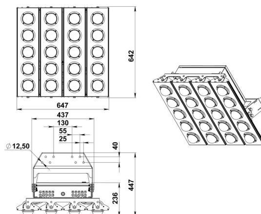
Габаритный чертеж
