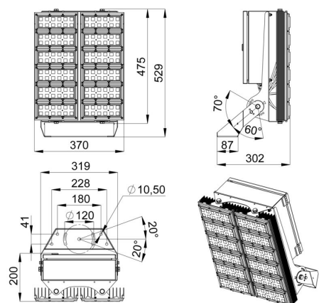
Габаритный чертеж
