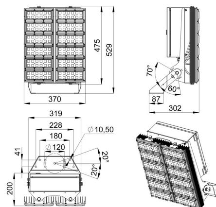
Габаритный чертеж
