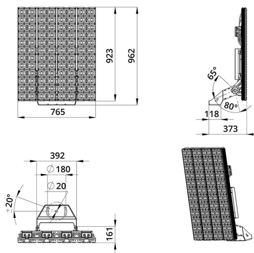
Габаритный чертеж
