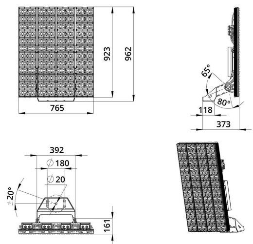
Габаритный чертеж
