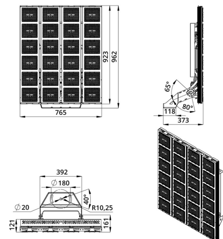
Габаритный чертеж
