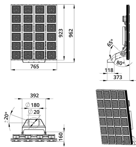
Габаритный чертеж
