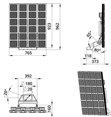
Габаритный чертеж
