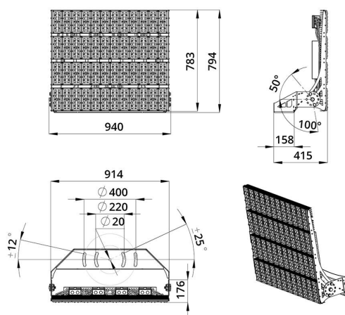
Габаритный чертеж
