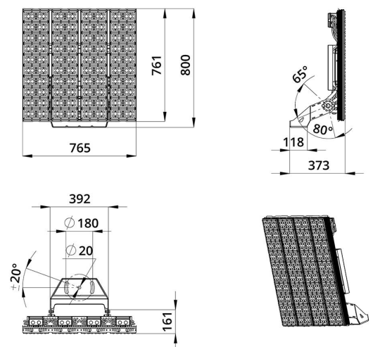
Габаритный чертеж
