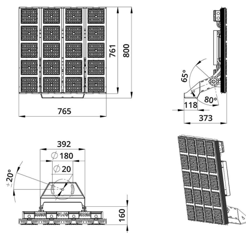
Габаритный чертеж
