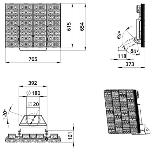
Габаритный чертеж
